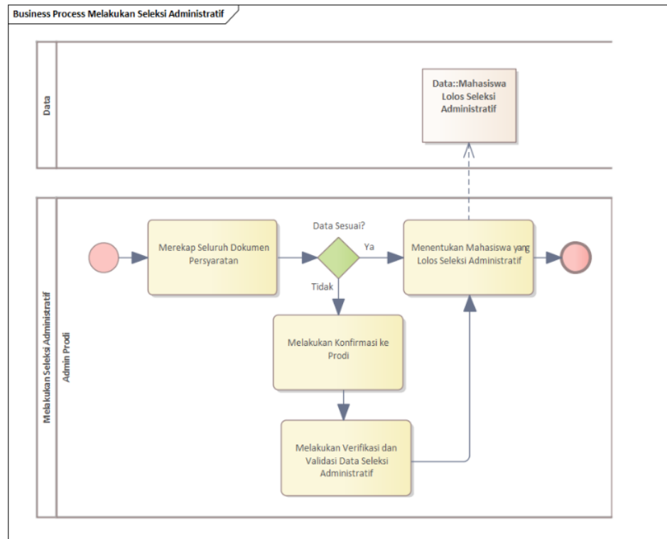
Gambar 10. Pemodelan proses seleksi adminsitrarif
