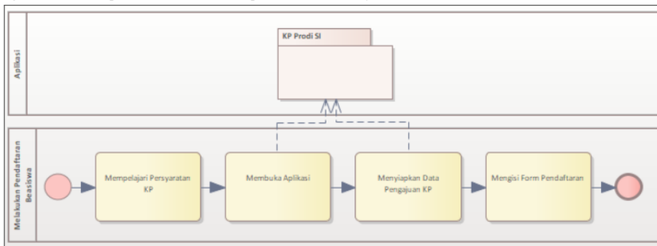
Gambar 8. Pemodelan Melakukan Pendaftaran KP
